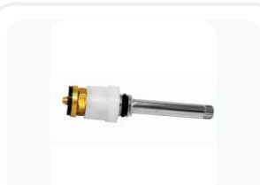
Reparo MVS CASTELO Registro1416DECA 1/2 e 3/4-204/224EixCromad
